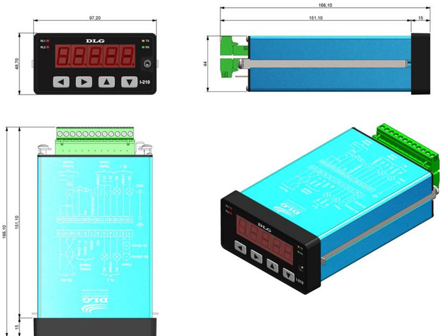
Figura 1 – Dimensionamento para montagem (cotas em milímetro)
