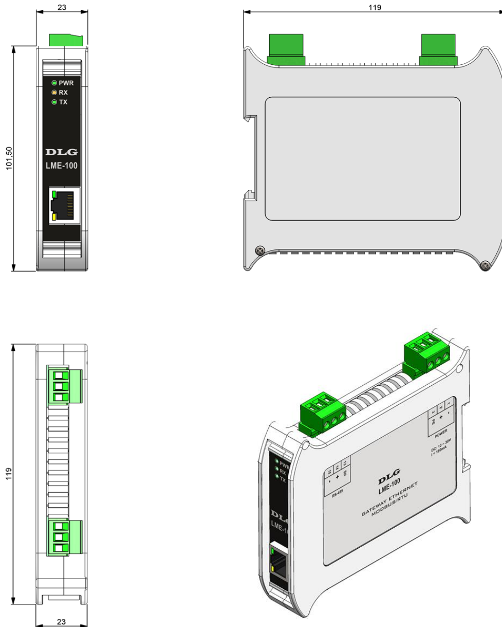
Figura 2 – Dimensionamento (Cotas em milímetro)
