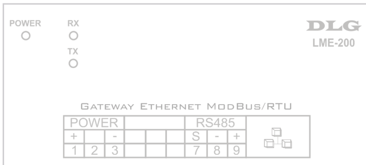
Figura 7 – Esquema da ligação elétrica na borneira traseira
