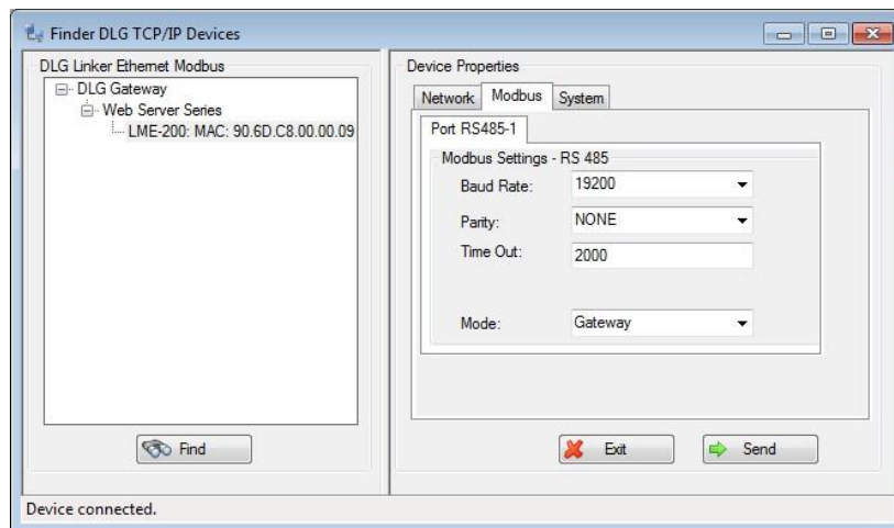
Figura 5 – Aba Modbus
