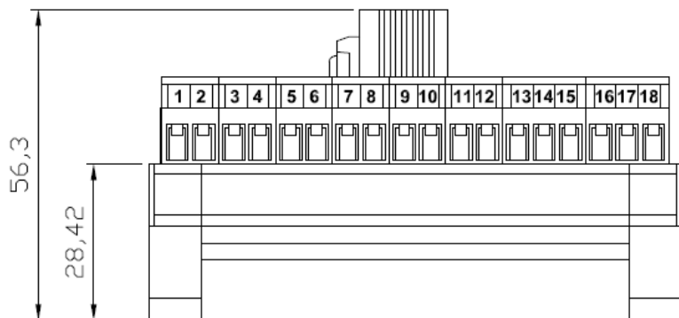
Vista Inferior
