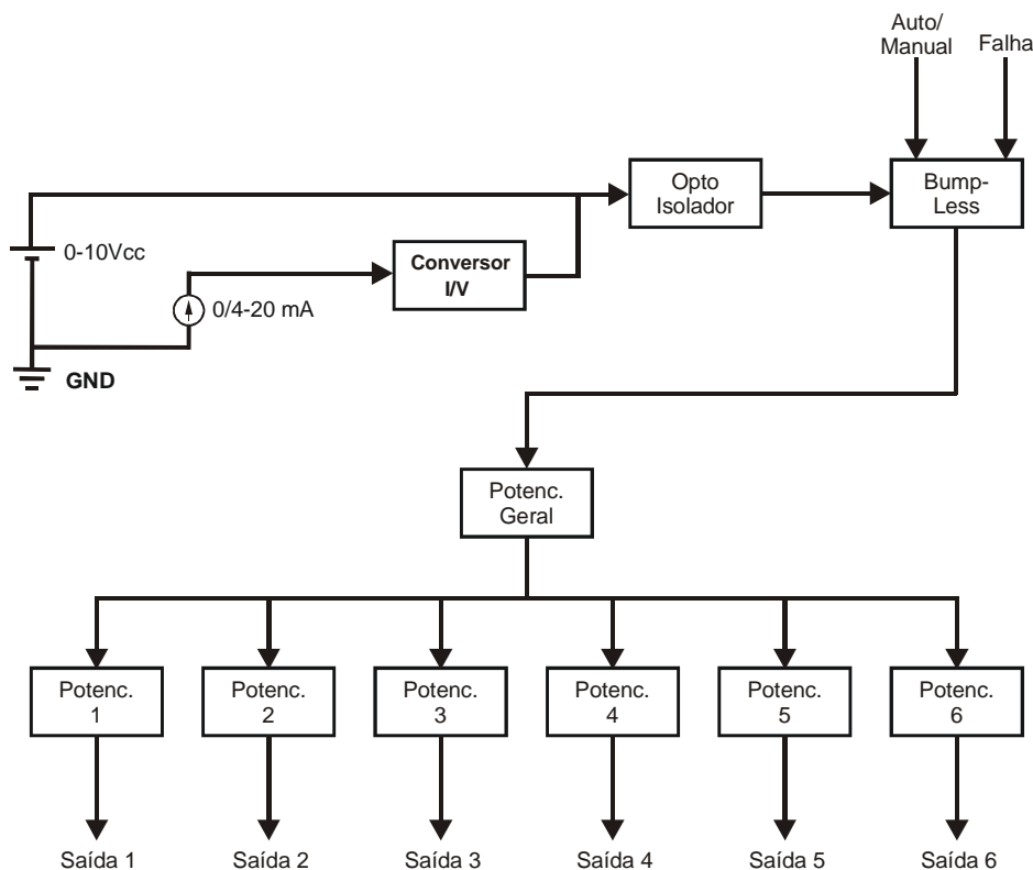
Figura 2 - Diagrama de Blocos Simplificado do SCV-700
