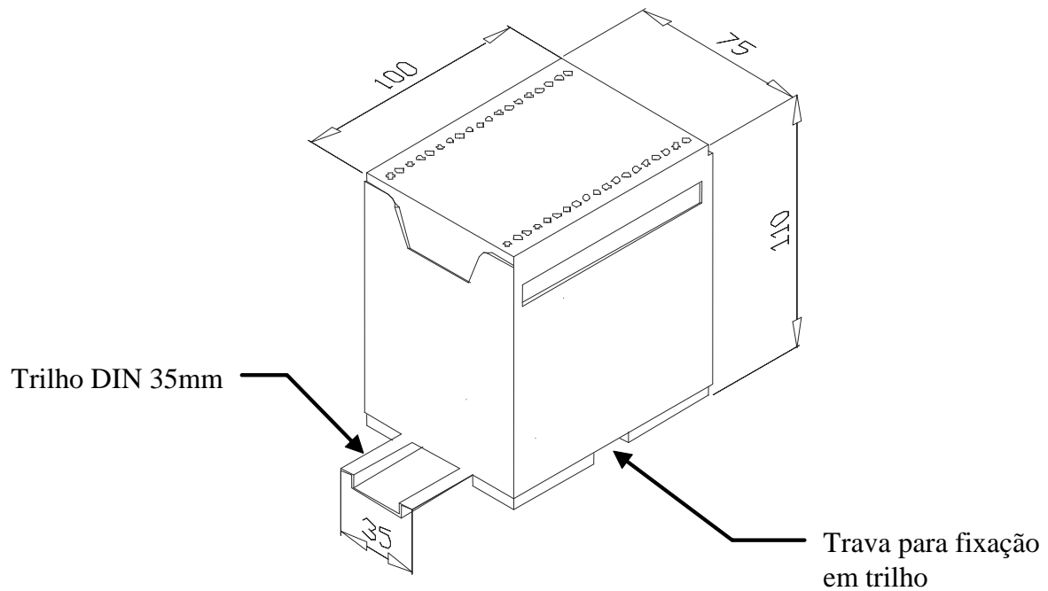
Figura 1 - Dimensões (em mm) do SCV700
