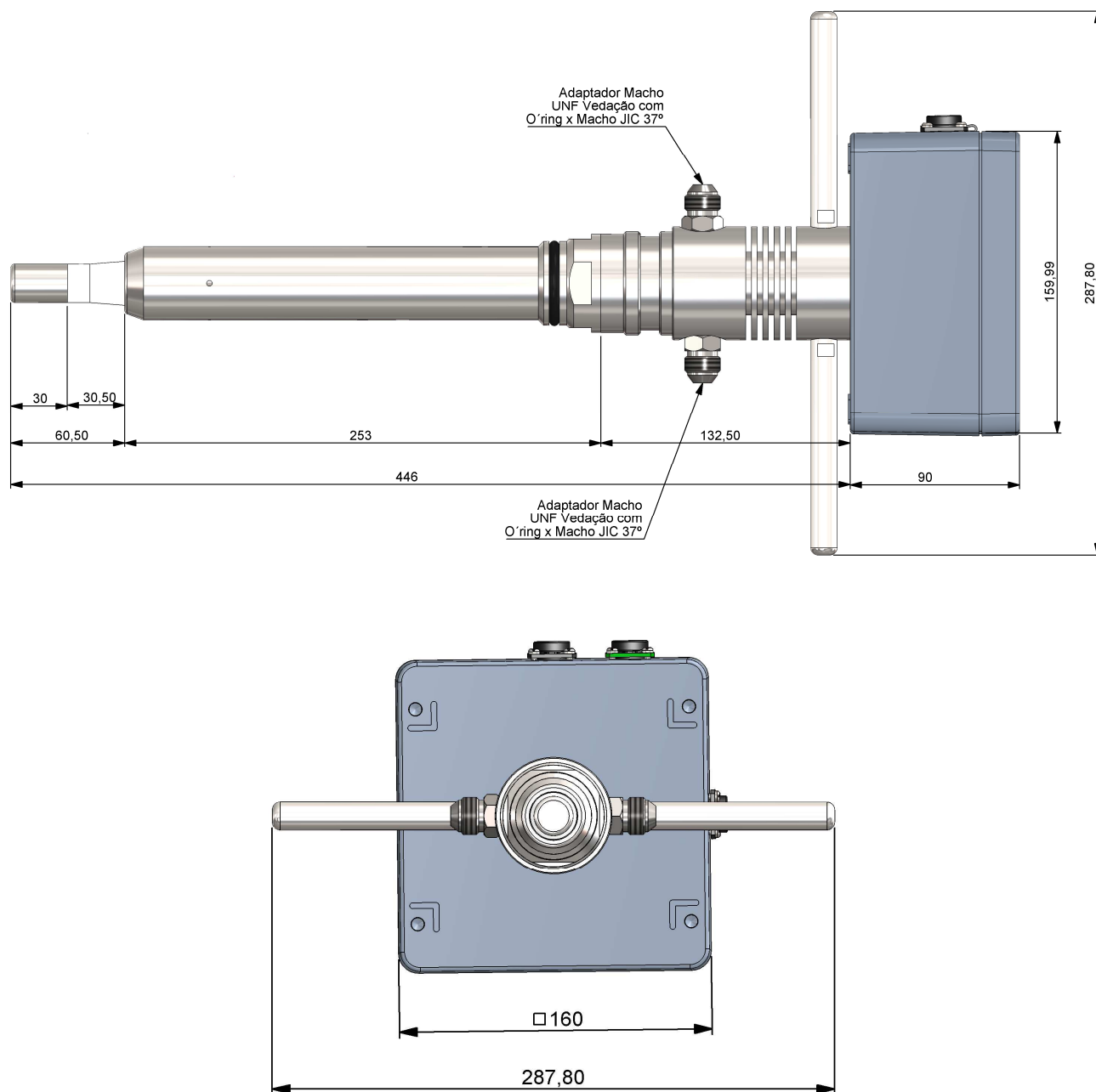
Figura 2 - Dimensionamento para montagem do Transmissor SD-3000/AL (Cotas em milímetro)
