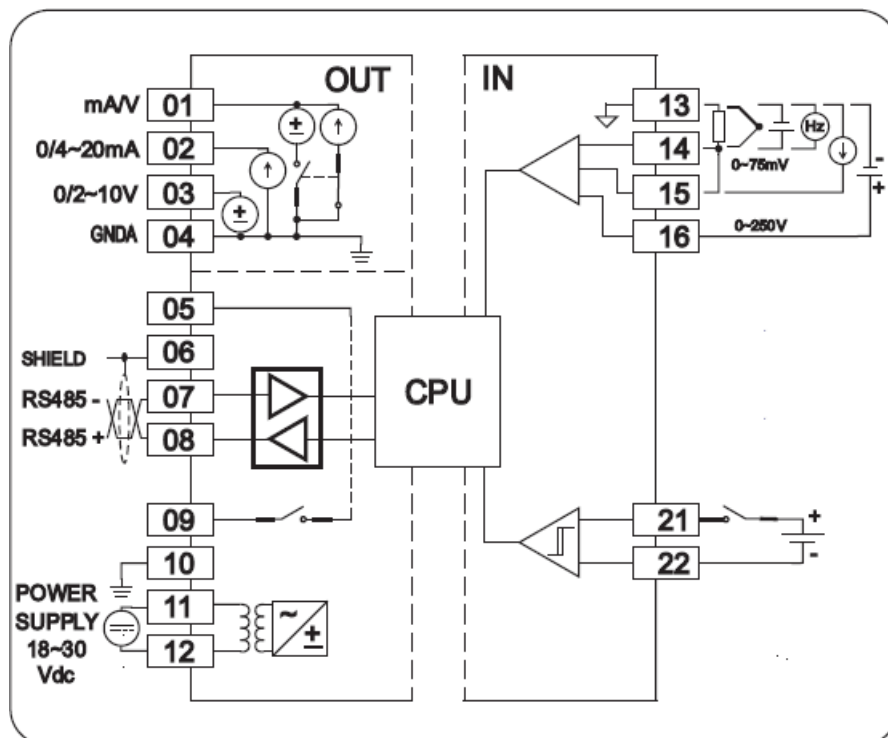
Diagrama geral da instalação elétrica XM-101 DC
