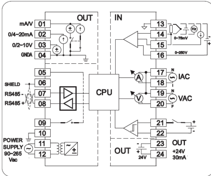
Diagrama geral da instalação elétrica da XM-101 AC
