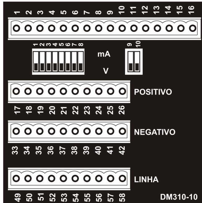
Figura 3 - Painel traseiro
