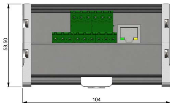
Figura 2 – Dimensionamento (Cotas em milímetro)
