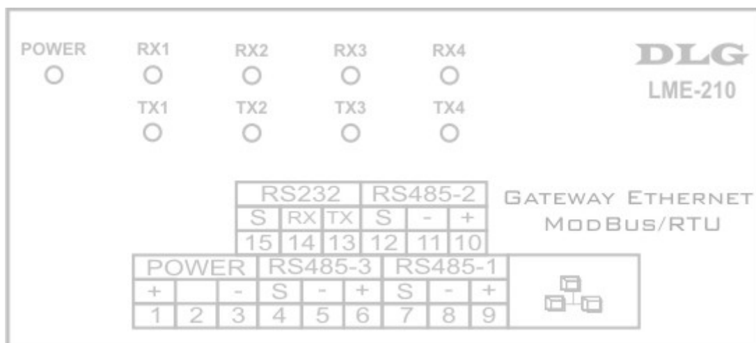
Figura 11 – Esquema da ligação elétrica na borneira traseira
