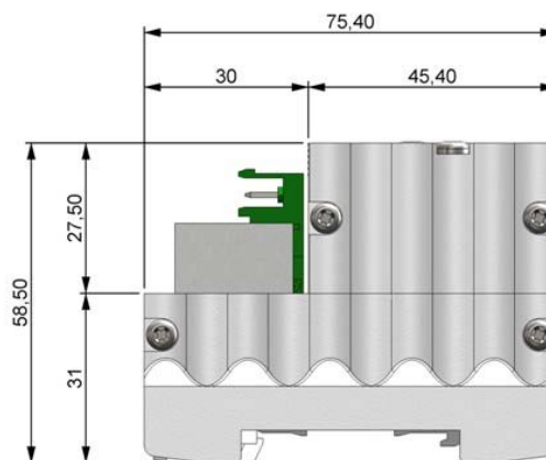
Figura 2 – Dimensionamento (Cotas em milímetro)
