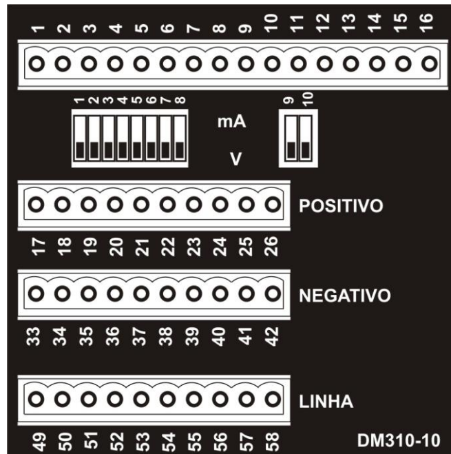
Figura 3 - Painel traseiro
