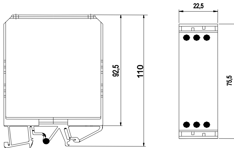
Figura 1 - Dimensionamento para montagem (Cotas em milímetro)
