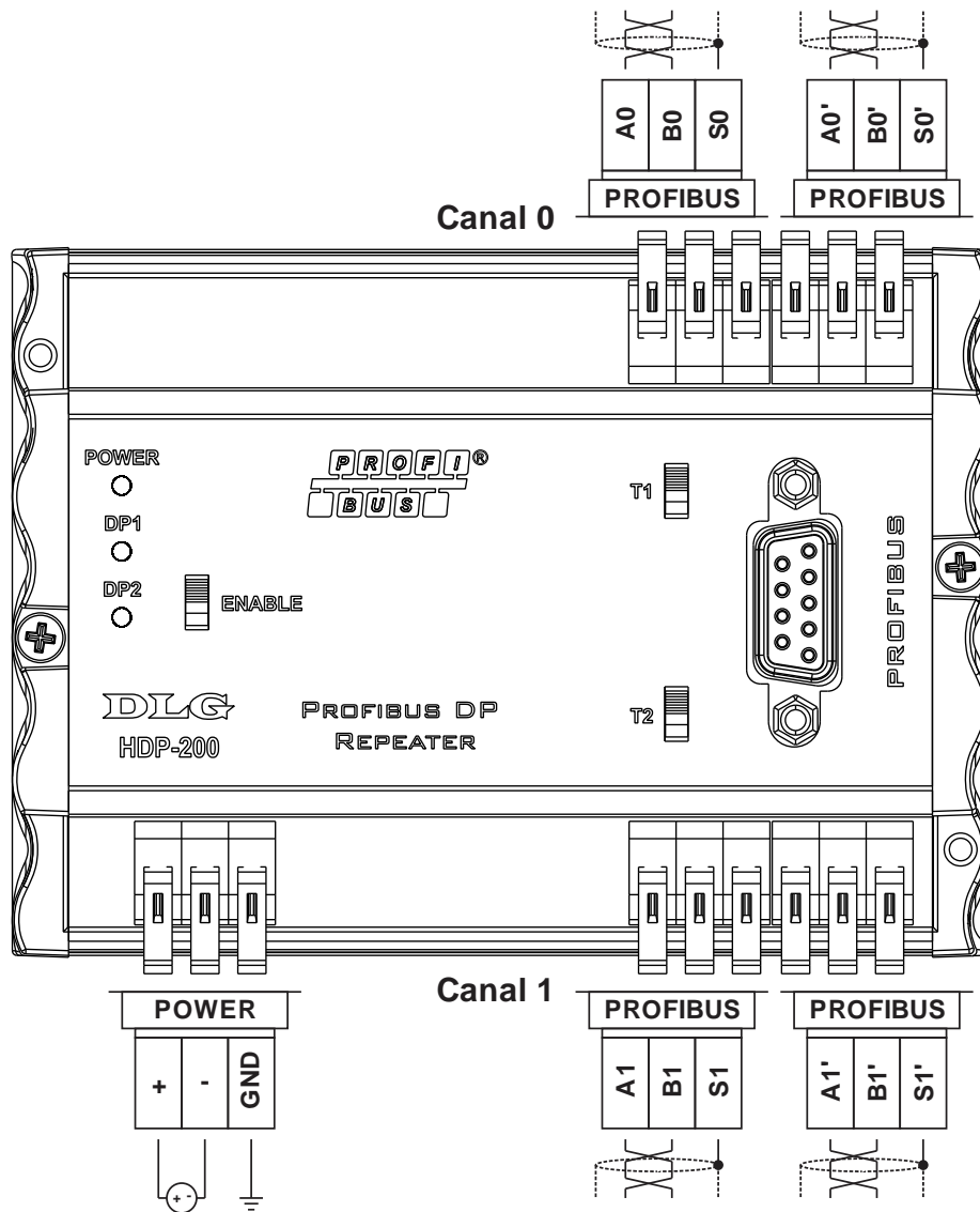
Figura 3 - Conexões elétricas do HDP-200.
