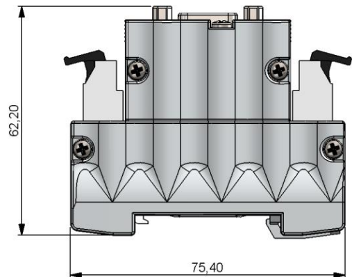
Figura 2 - Dimensionamento para montagem (cotas em milímetros)
