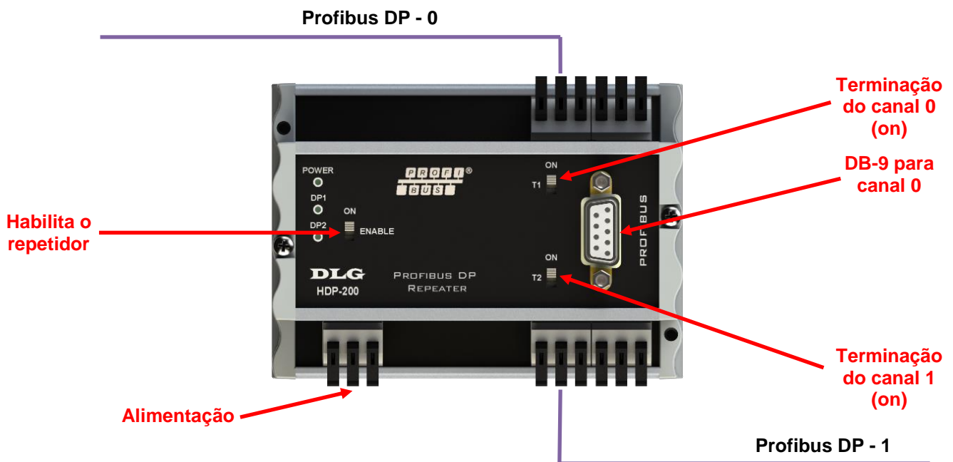
Figura 5 – Instalação com terminação
