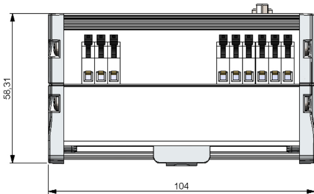
Figura 2 - Dimensionamento para montagem (cotas em milímetros)
