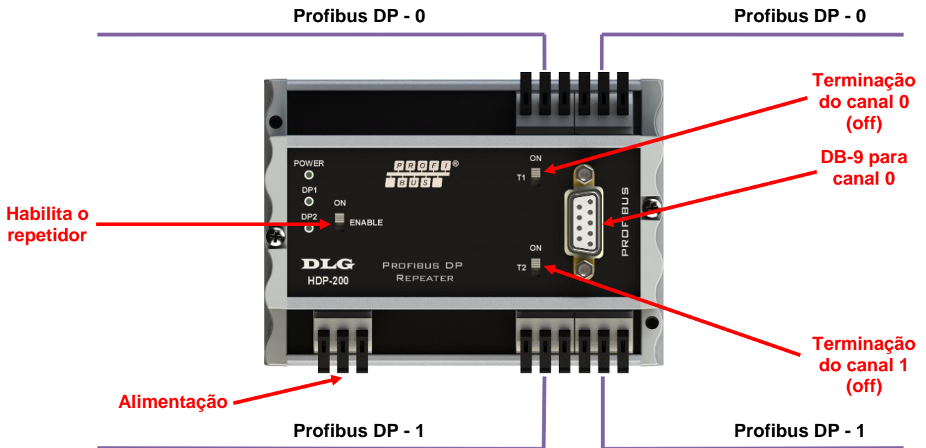
Figura 4 – Instalação sem terminação
