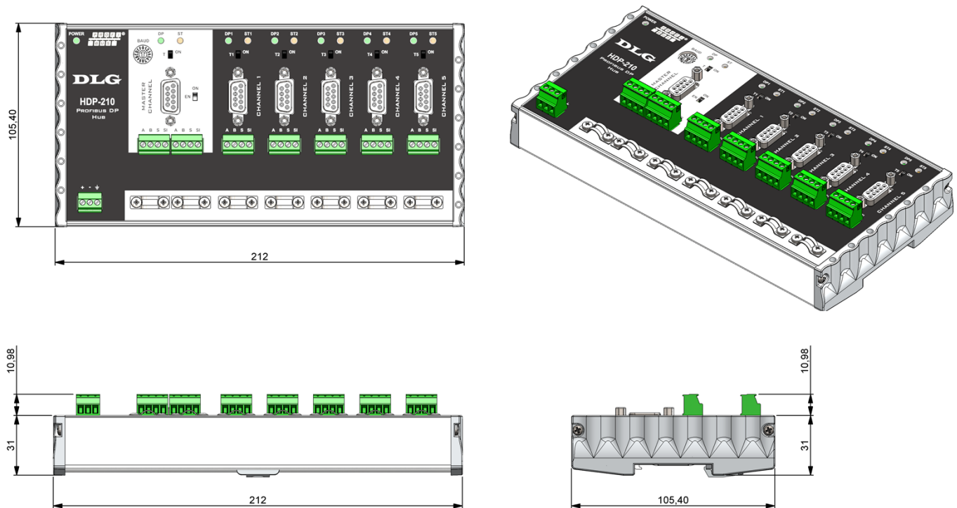
Figura 2 - Dimensionamento para montagem (cotas em milímetros)
