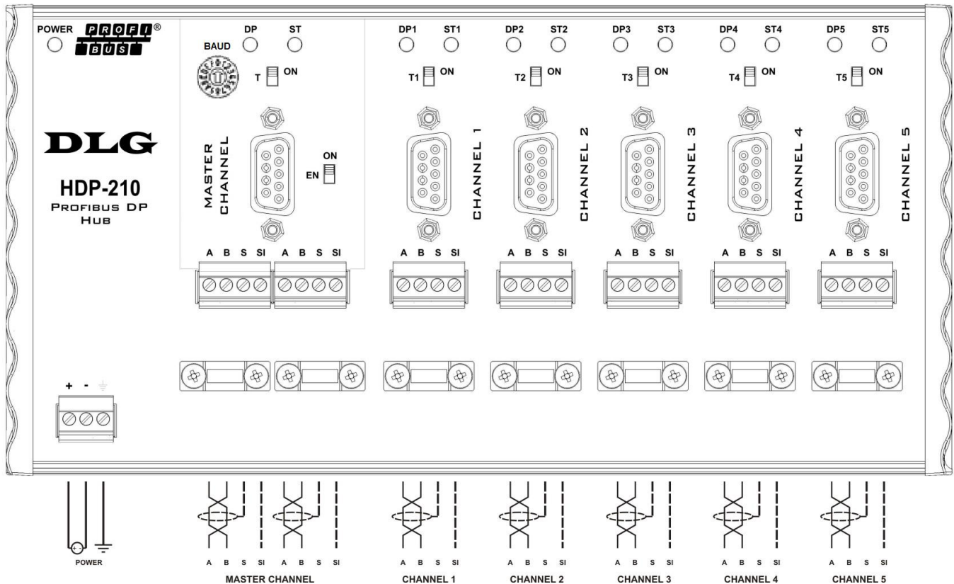
Figura 3 - Conexões elétricas do HDP-210.
