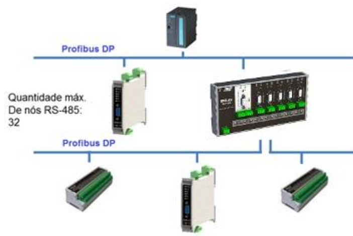
Figura 1 - Aplicação do HDP-210.
