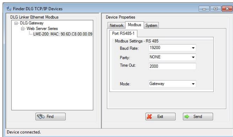
Figura 5 – Aba Modbus
