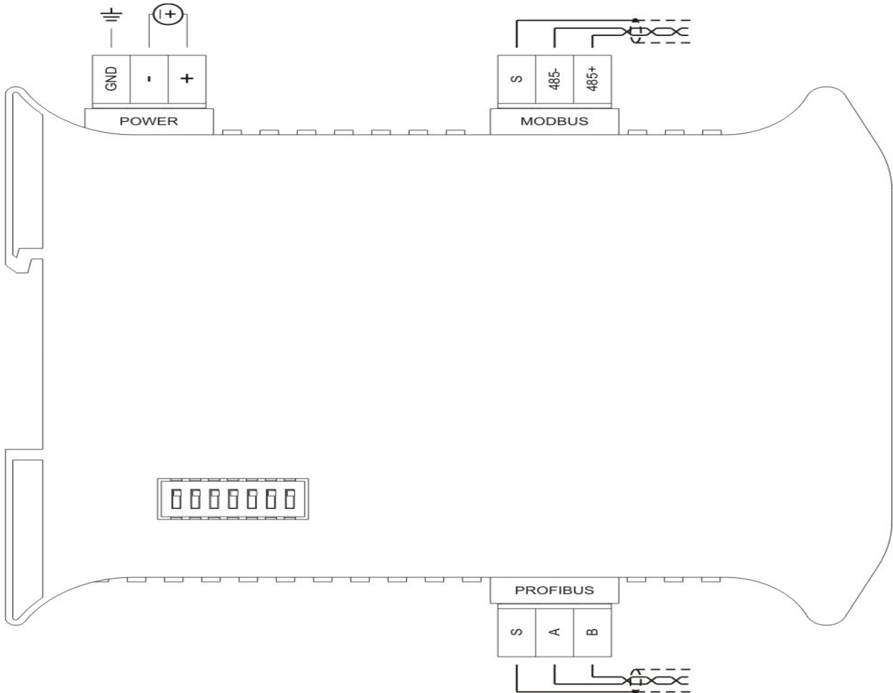
Figura 3 - Conexões elétricas do LMP-100.
