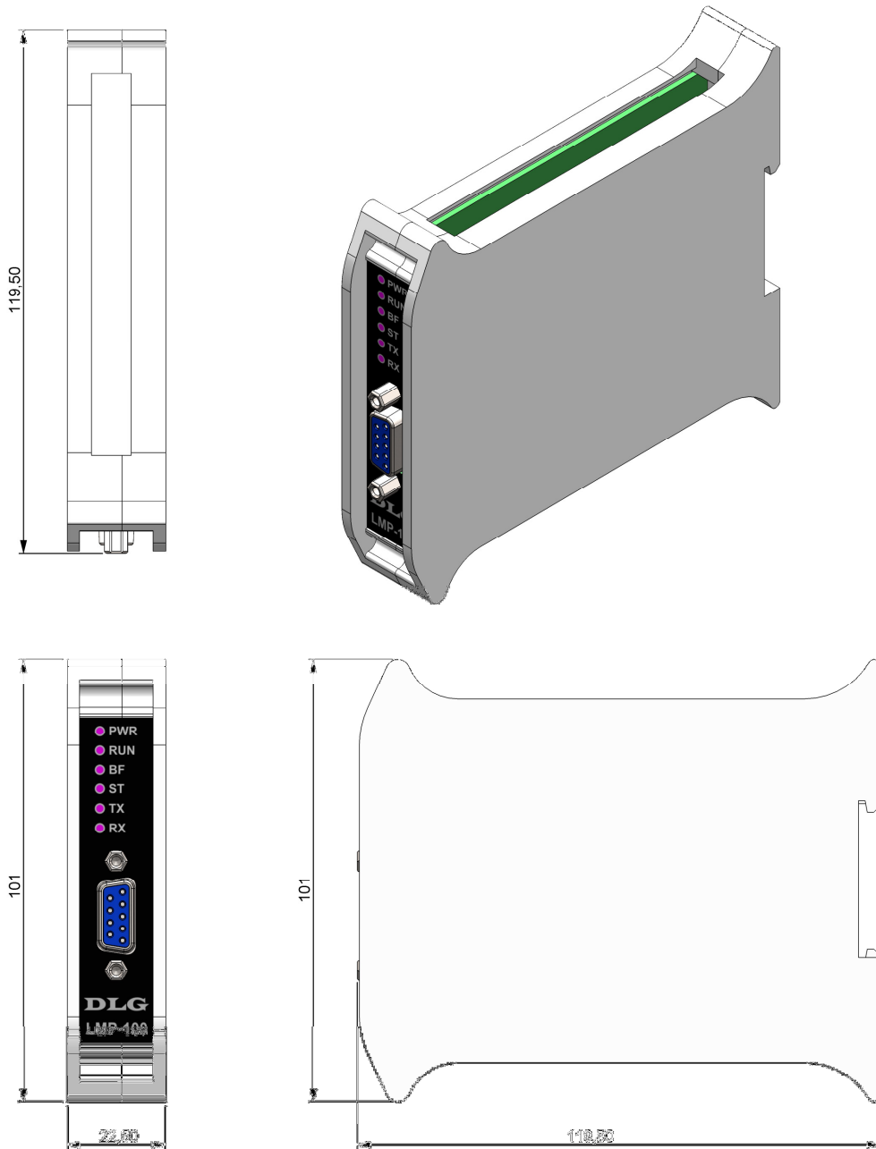
Figura 2 - Dimensionamento para montagem (cotas em milímetros)
