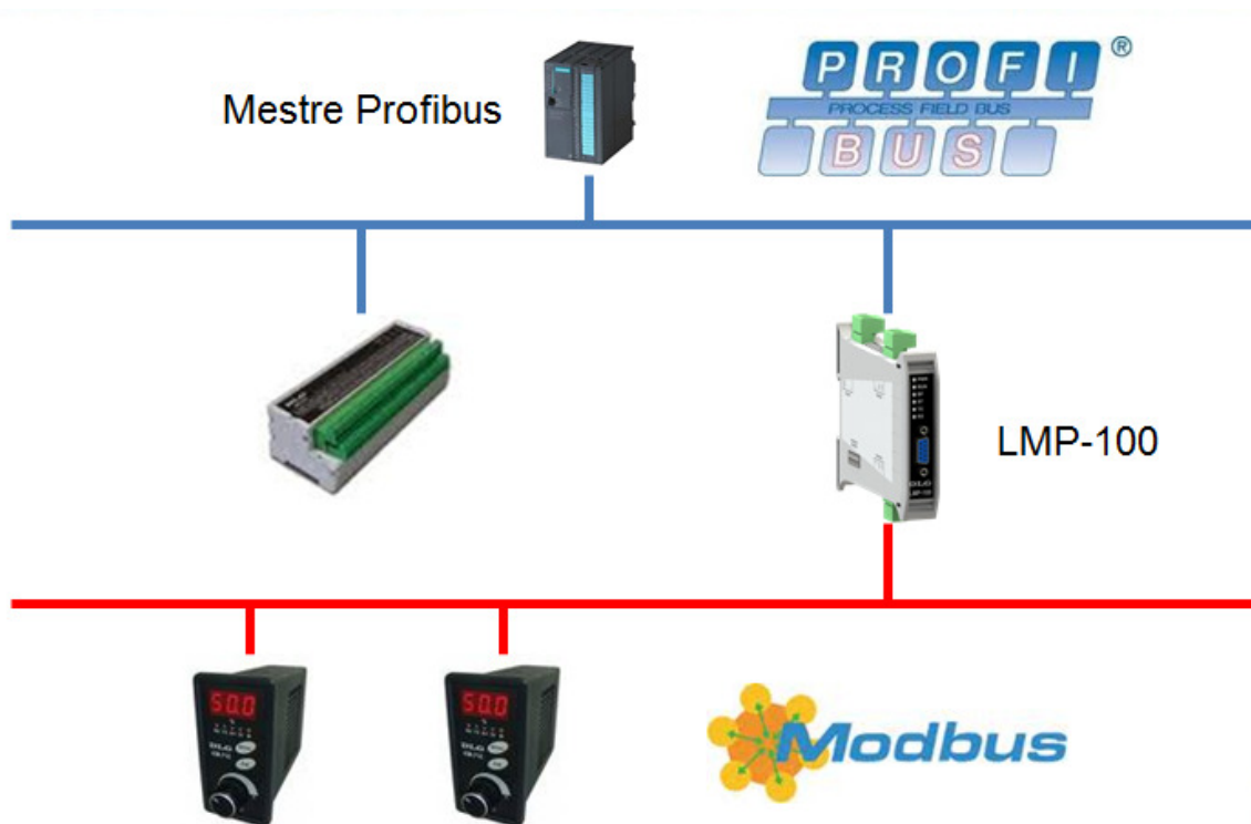
Figura 1 - Aplicação do LMP-100.
