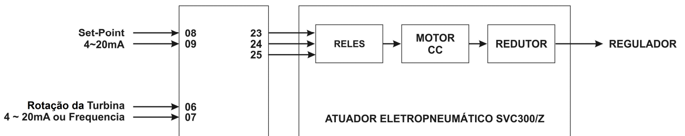
Figura 6 - Resumo esquemático do PSM-750A/Z
