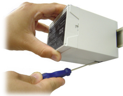
Traseira do conversor com encaixe para trilho
