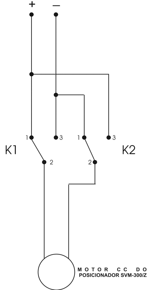
Figura 9 - Ligação dos contadores para o PSM-750A/Z
