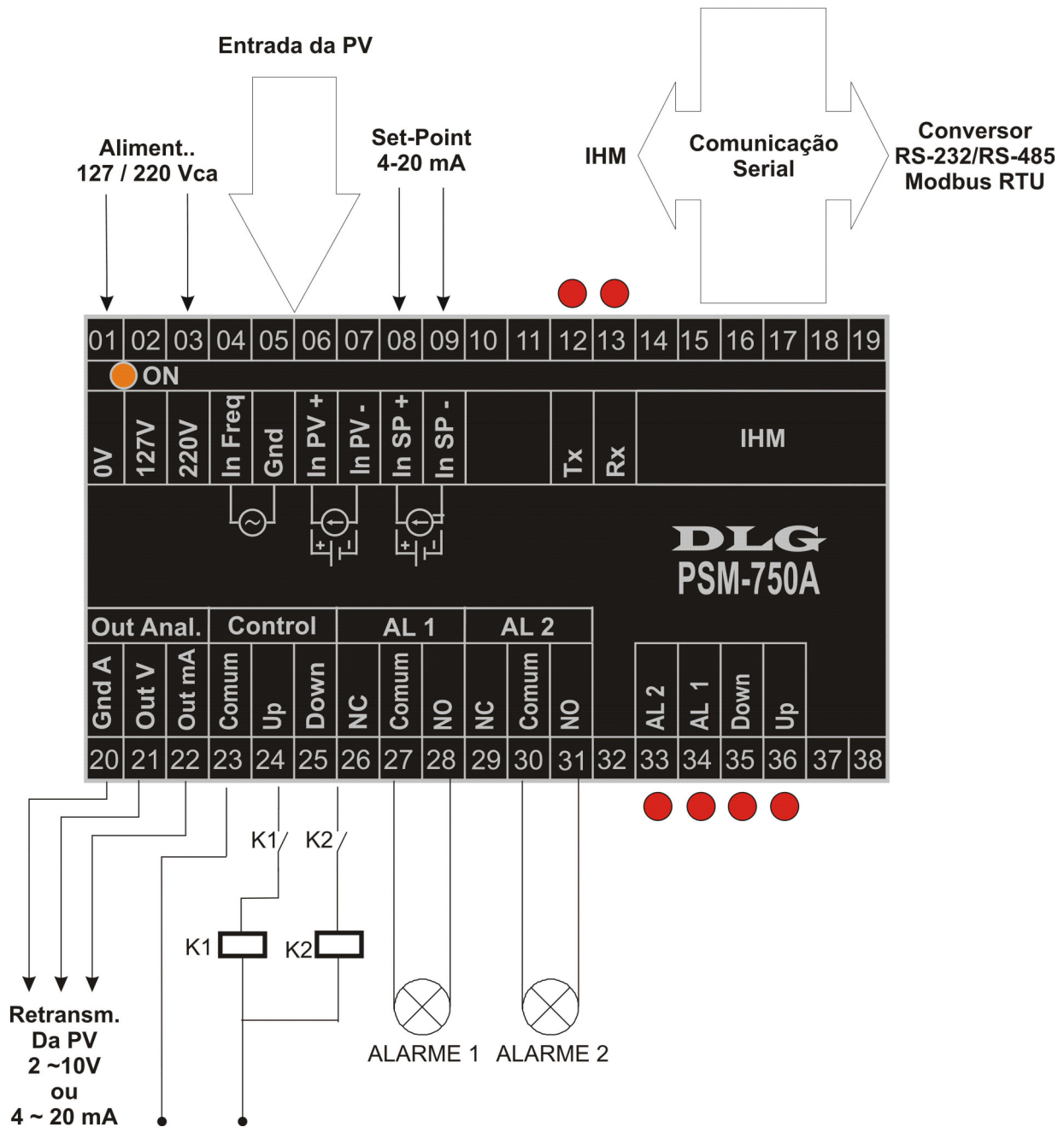
Figura 2 - Ligação do PSM-750A com alimentação 127/220Vca
