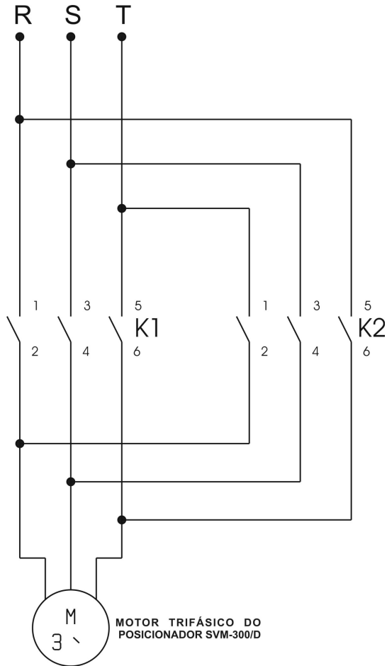
Figura 8 - Ligação dos contadores para o PSM-750A/D
