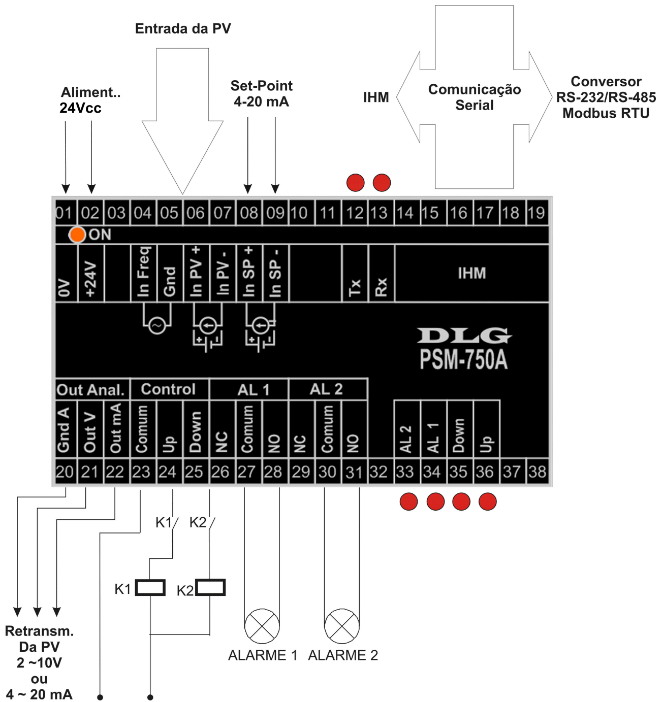
Figura 3 Ligação do PSM-750A com alimentação 24Vcc
