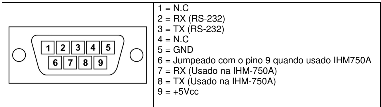
Figura 12 - Disposição dos pinos do DB-9 do PSM-750A
