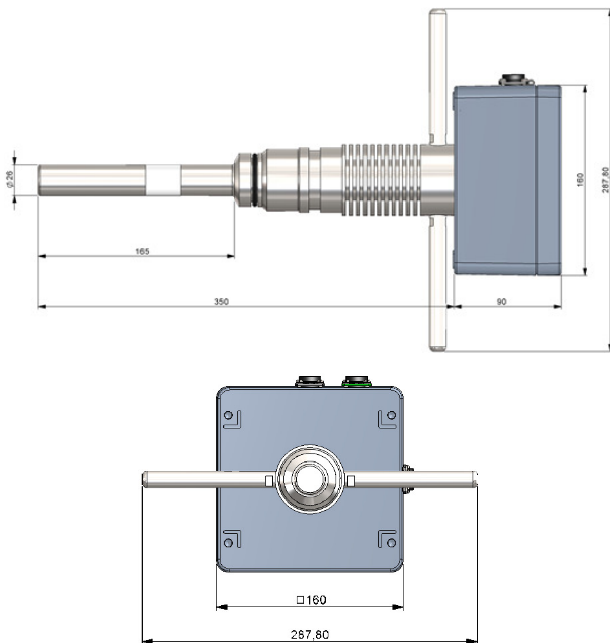
Figura 1 - Dimensionamento para montagem do Transmissor SD-3000 (Cotas em milímetro)
