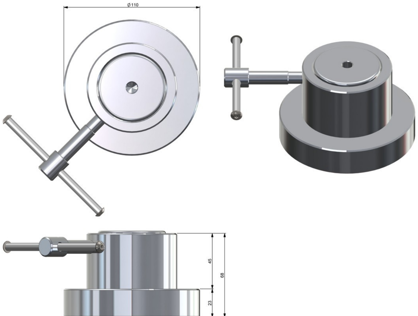
Figura 3 - Dimensionamento para montagem do Flange (Cotas em milímetro)
