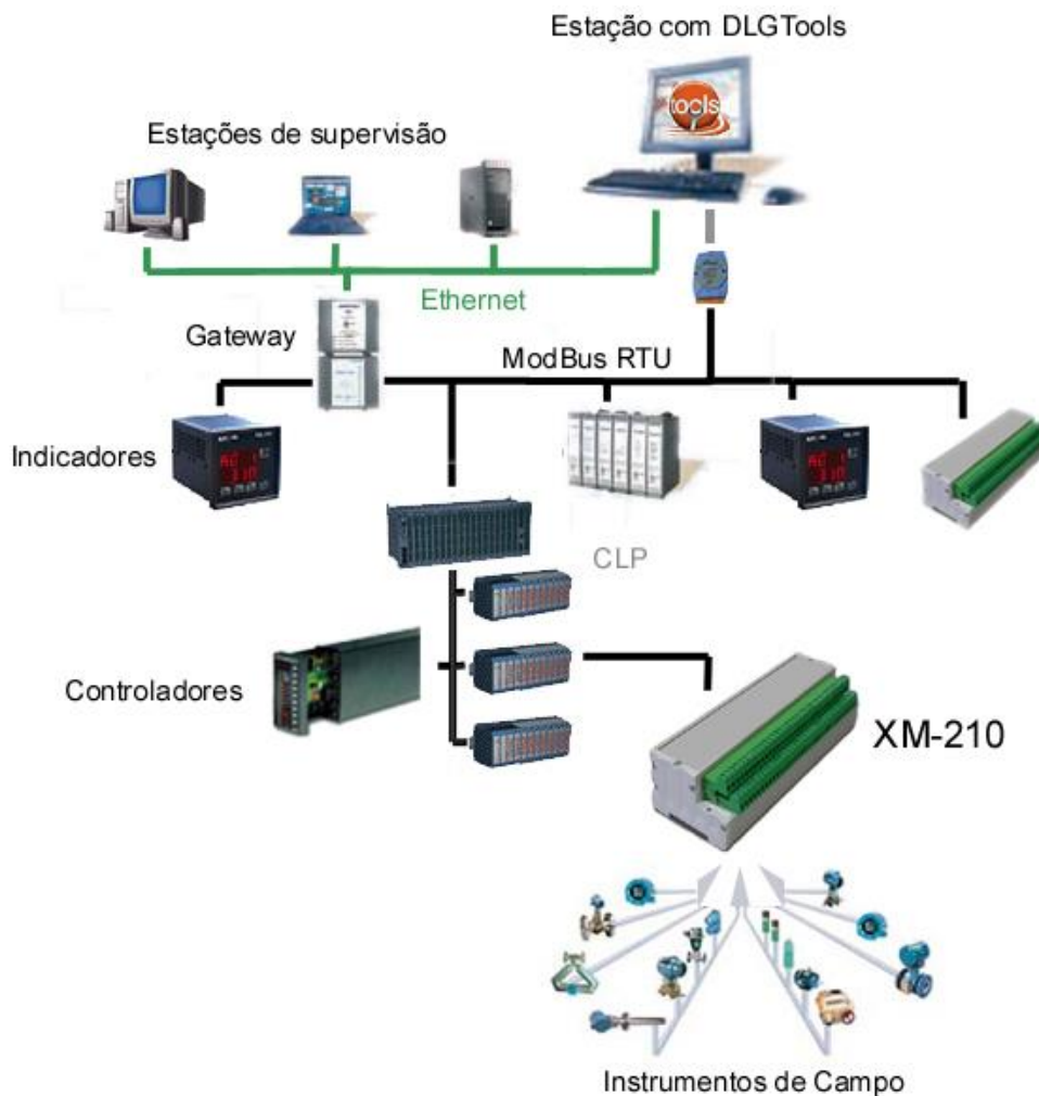
Figura 2 – Topologia rede Modbus com a XM-210
