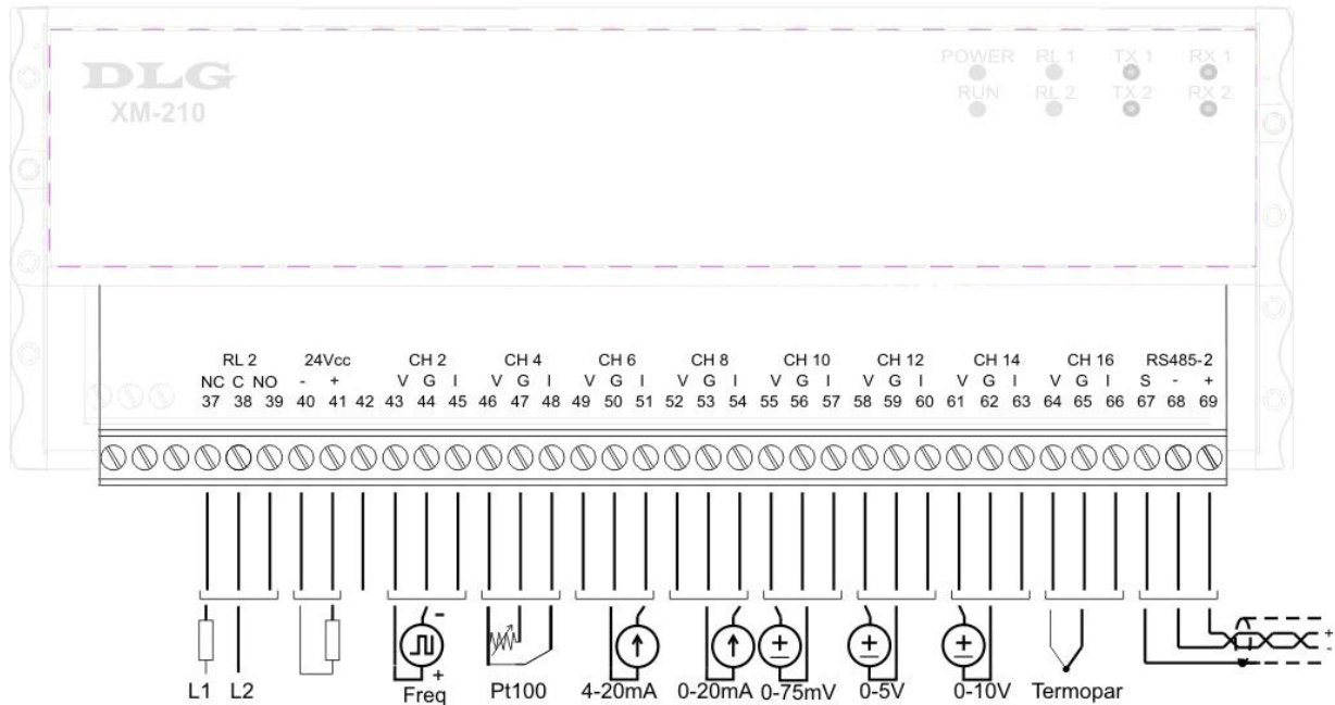
Figura 8 Borneira Inferior
