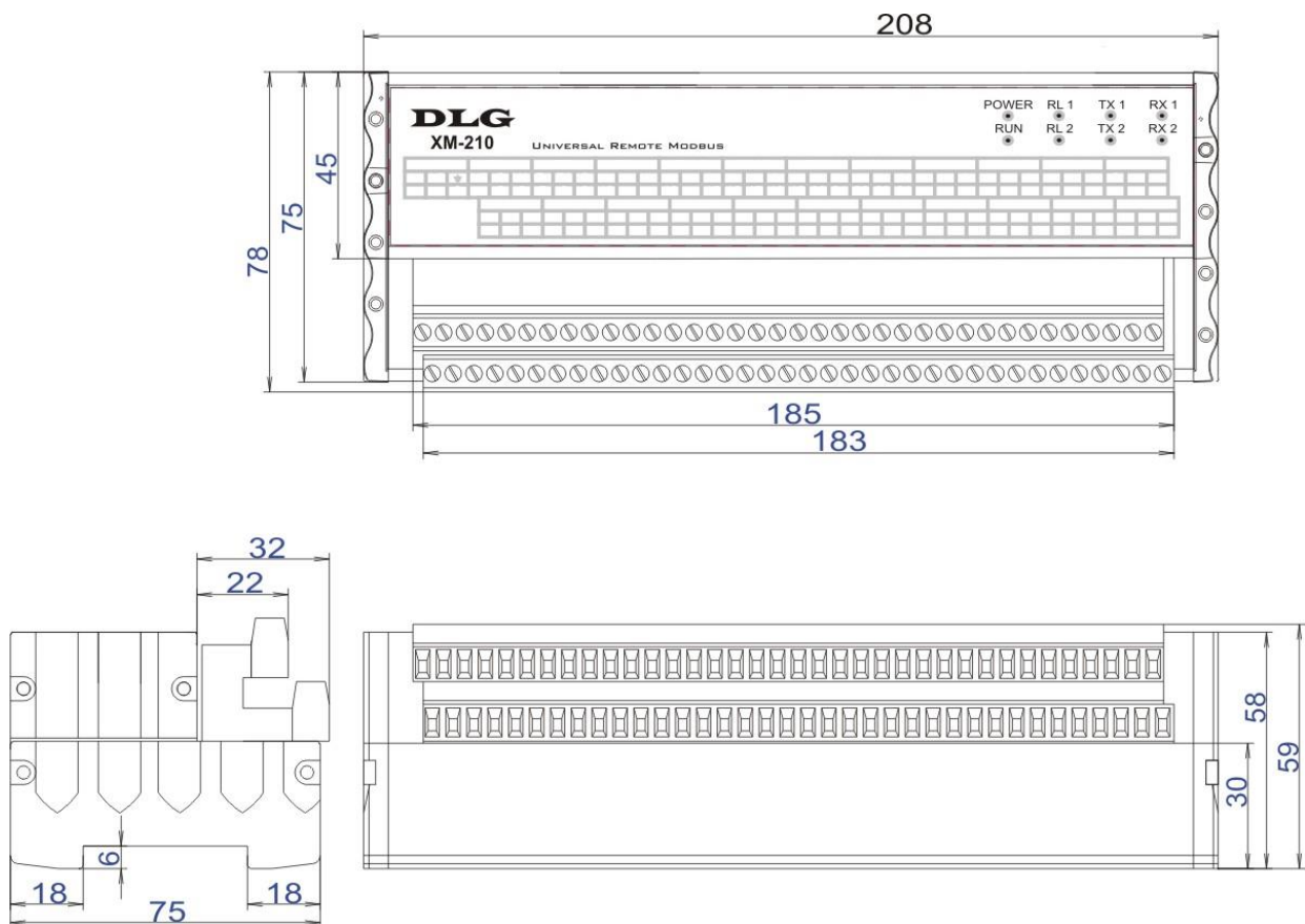
Figura 3 – Dimensionamento para montagem (Cotas em milímetros)
