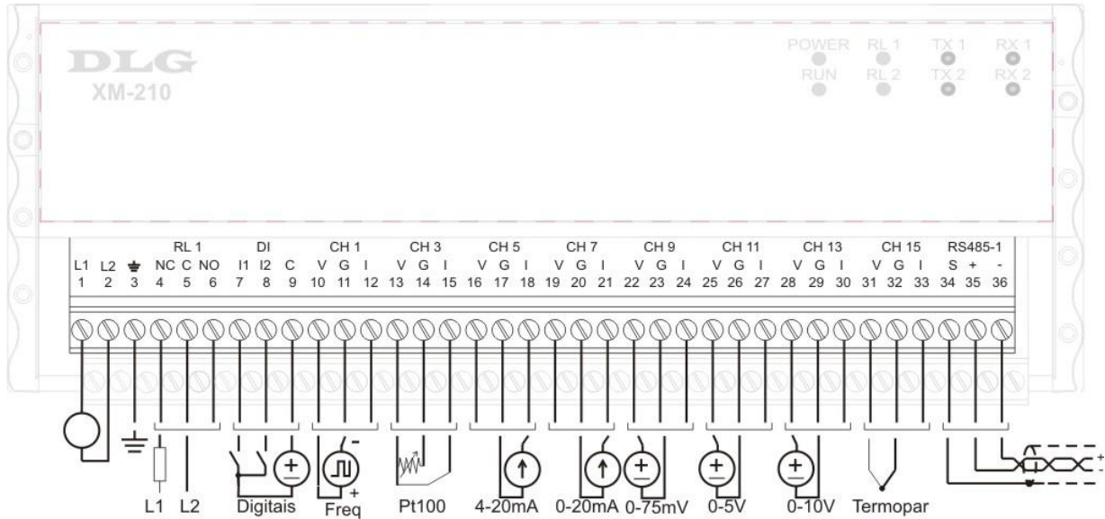
Figura 7 Borneira Superior
